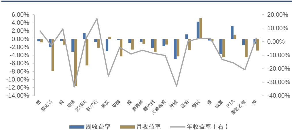
图 2.1：南华工业品指数品种指数近期收益图
