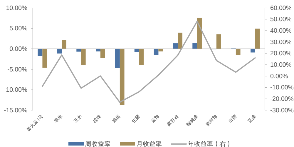
图 2.4：主要商品指数近期收益图
