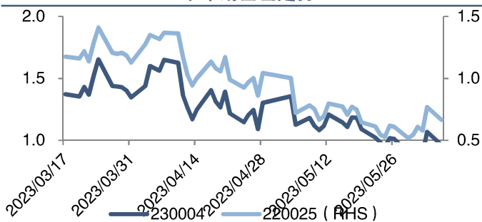
十年期基差走势
