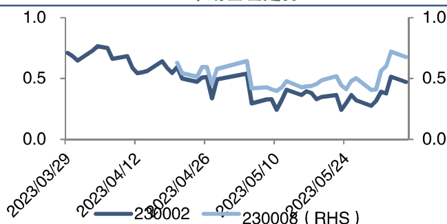
三十年期基差走势
