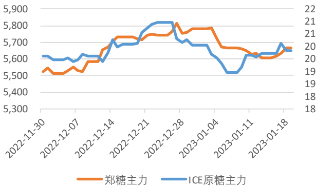
内外盘对照
