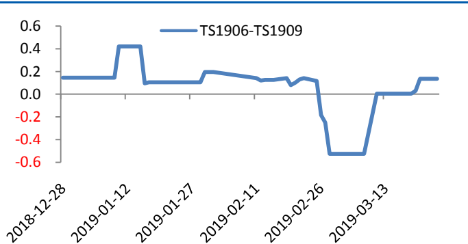
图6 TS合约跨期价差
