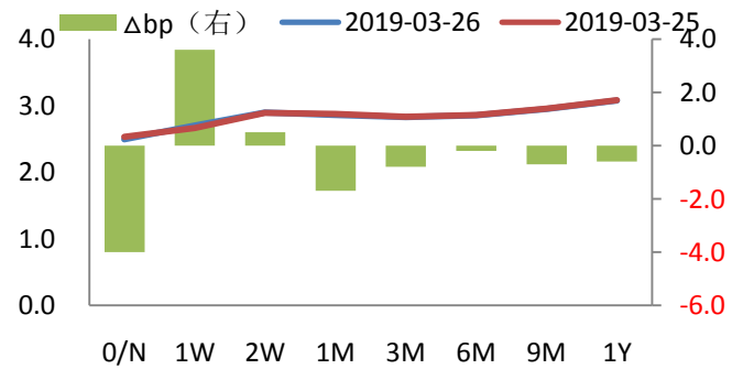
图 16 Shibor 利率日变动
