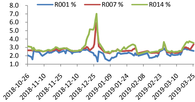
图 13 银行间质押式回购利率变动
