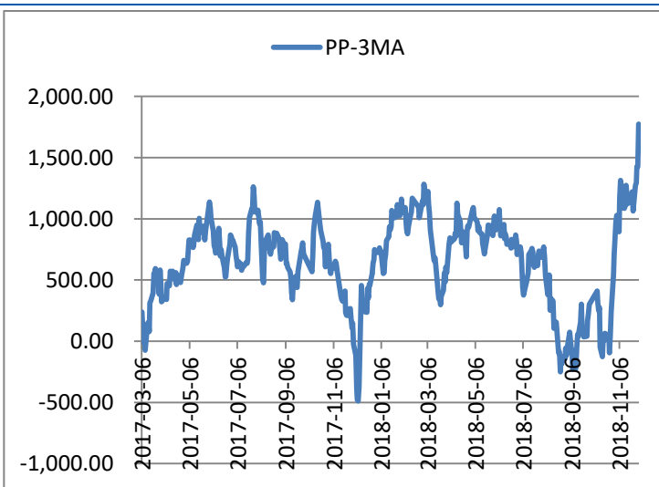
PP-3MA 价差
