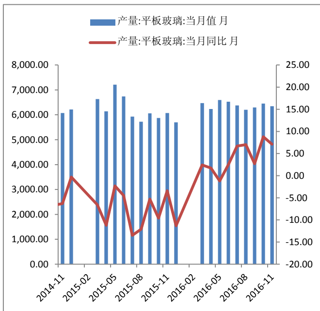
图 3：玻璃产量
