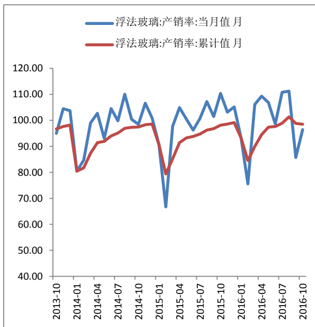
图 4：玻璃产销率
